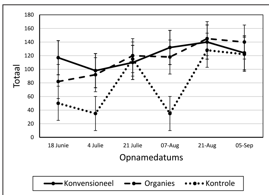
FIGUUR 5: Voedingsaktiwiteit gemeet met aaslamina op die konvensionele, organiese en kontrolepersele op die verskillende opnatedatums tussen Junie en September [datum*behandeling; LS Gemiddeld; Effek: F(10.30) = 2.6975 , p = 0.1730 . Vertikale kolomme – betroubaarheidsvlak 0.95]
